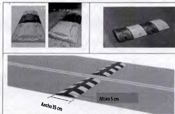
Figura 4. Especificaciones Resalto portátil
