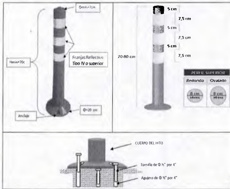
Figura 3 Delineador tubular.
